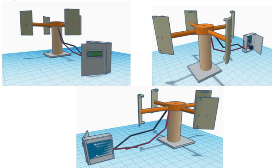
Gambar 4 Perancangan Mekanik
