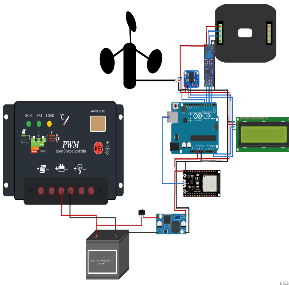
Gambar 3 Perancangan Elektronika
