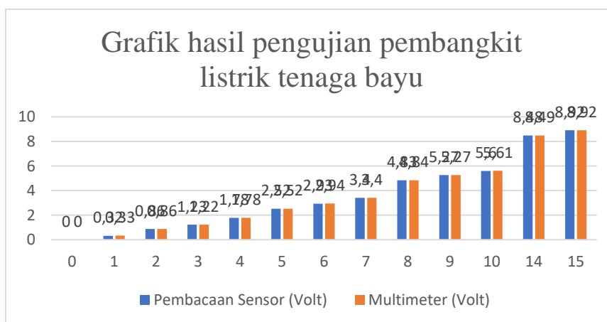
Gambar 8 Grafik Hasil pengujian pembangkit listrik tenaga bayu
