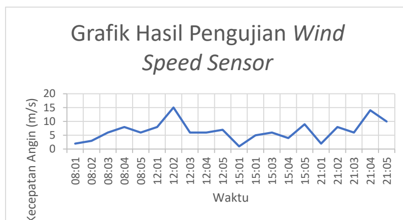
Gambar 6 Grafik Hasil Pengujian Wind Speed Sensor
