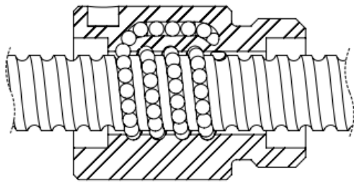
Gambar 2. Penampang Potong Poros berulir [5]
