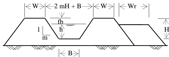
Gambar 1. Bentuk penampang saluran di daerah timbunan
