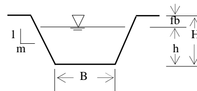
Gambar 3. Penampang saluran primer dan sekunder
