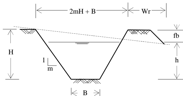
Gambar 2. Bentuk penampang saluran di daerah galian
