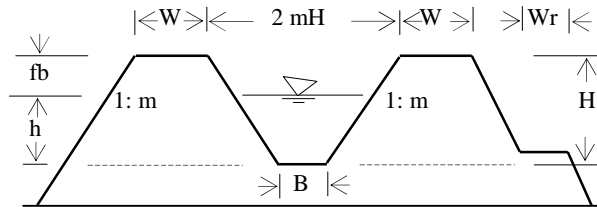
Gambar 4. Bentuk penampang saluran tersier-kuarter
