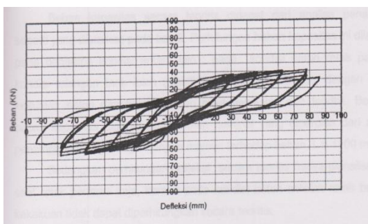
Gambar 6 . Grafik Beban – Defleksi Percobaan Siklik 3
