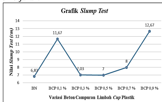
Gambar 3.1 Hasil Pengujian Slump Beton
