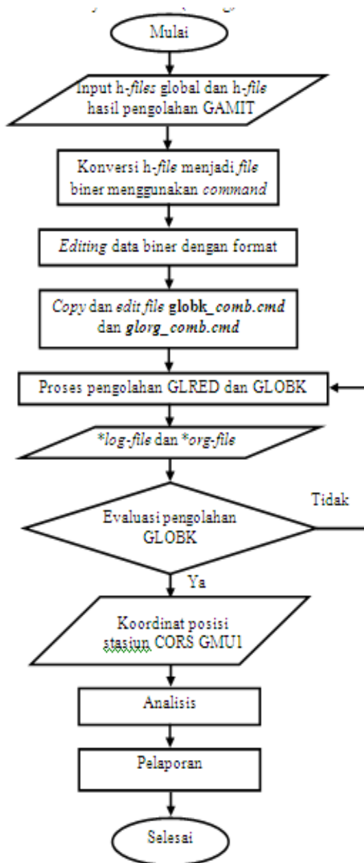
Gambar 2. Pengolahan dengan GLOBK
