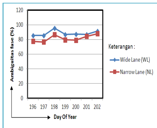
Gambar 4. Nilai WL dan NL
