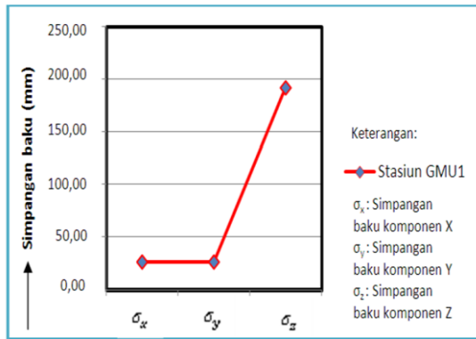
Gambar 8. Nilai simpangan baku koordinat stasiun GNSS CORS GMU1
