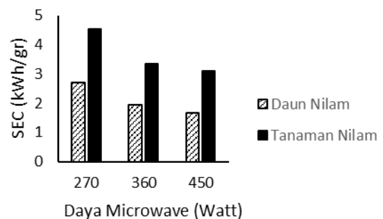
Gambar 4. Nilai (SEC) pada Metode Microwave Hydrodistillation
