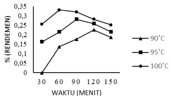
Gambar 3. Pengaruh Variasi Temperatur dan Waktu distilasi terhadap rendemen minyak daun nilam
