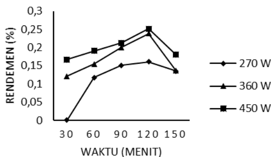
Gambar 2. Pengaruh Daya dan Waktu Terhadap Jumlah Produk dalam % Rendemen
