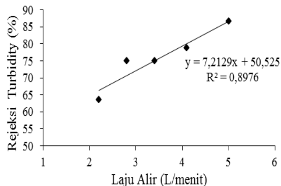
Gambar 7 Grafik Pengaruh Laju Alir terhadap % Rejeksi Kekekruhan pada RO.
