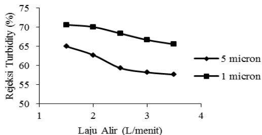
Gambar 6 Pengaruh Laju Alir terhadap % Rejeksi Kekekruhan pada Mikrofiltrasi.
