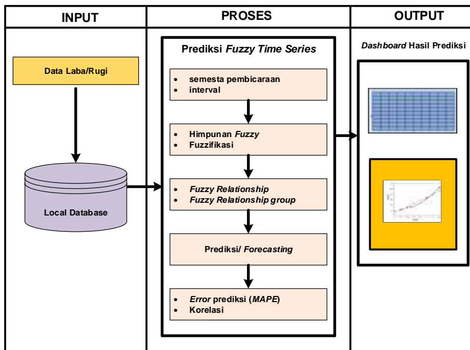
Gambar 1 Kerangka sistem informasi
