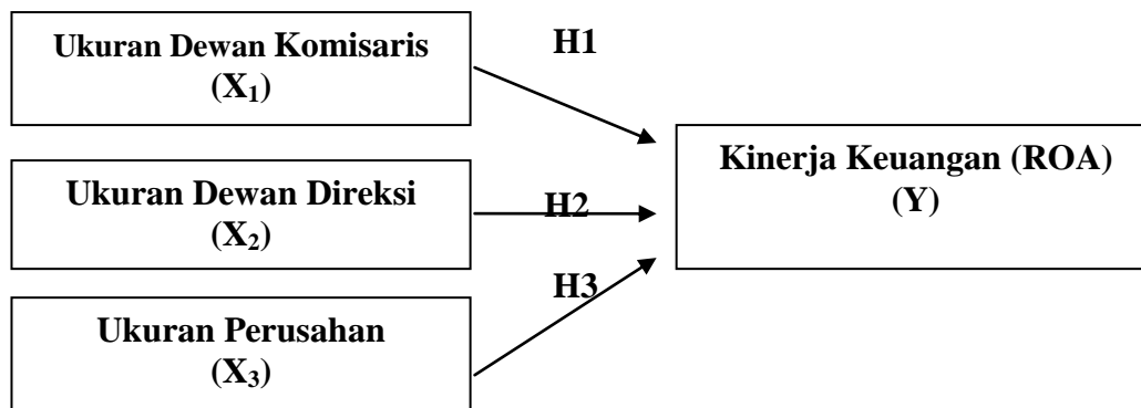
Gambar 2. Kerangka Pemikiran
