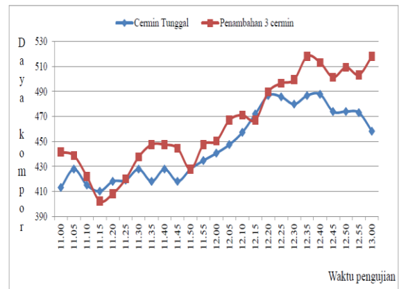
Grafik 5. Daya Kompor Surya
