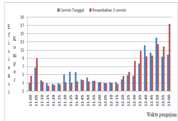
Grafik 6. Efisiensi Kompor Surya
