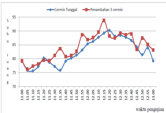
Grafik 4. Kenaikan Temperatur Air Dalam Kompor Kotak
