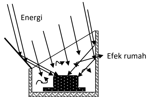
Gambar 1. Distribusi Energi Panas Di Dalam Kompor
