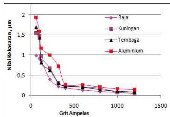
Gambar 7 : Grafik Capaian Kekasaran Tiap Grit Ampelas
