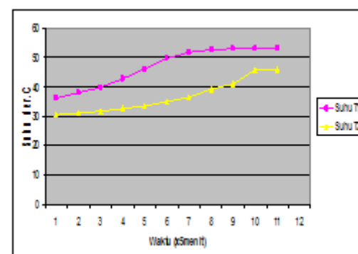
Gambar 11. Grafik Hubungan waktu dan Suhu Pengeringan Baju Kaos
