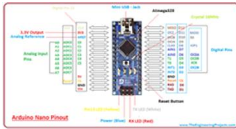
Gambar 1 Arduino Nano
