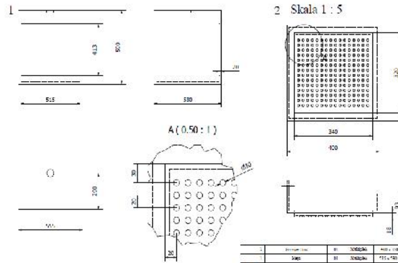
Gambar 3. Kerangka Alat Vacuum Box dan Meja
