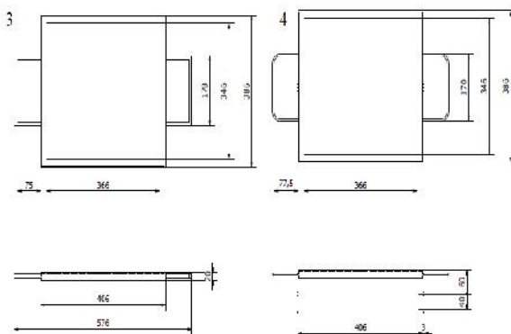
Gambar 4. Kerangka Alat Clamp Lower dan Clamp Upper
