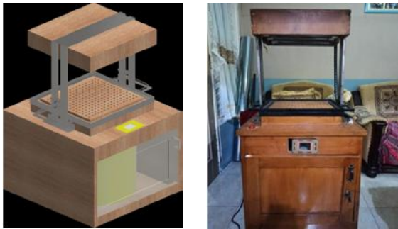
a. Desain b. Hasil Rancang Bangun Gambar 5. Alat Vacuum Forming
