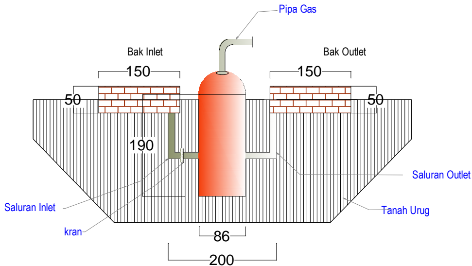
Gambar 4. Instalasi reaktor biogas
